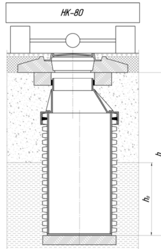
Расчётная схема:
