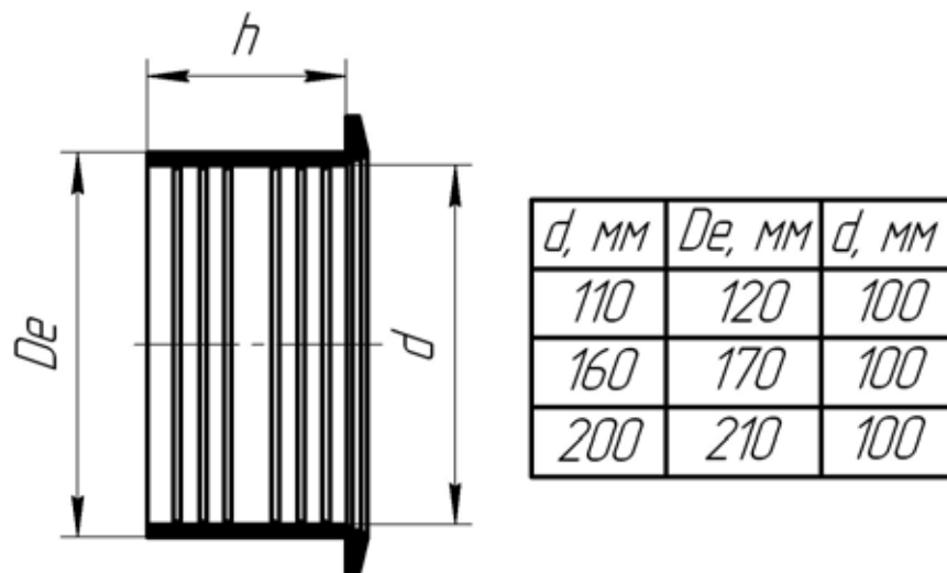
Рис. 43. Уплотнительная манжета.
