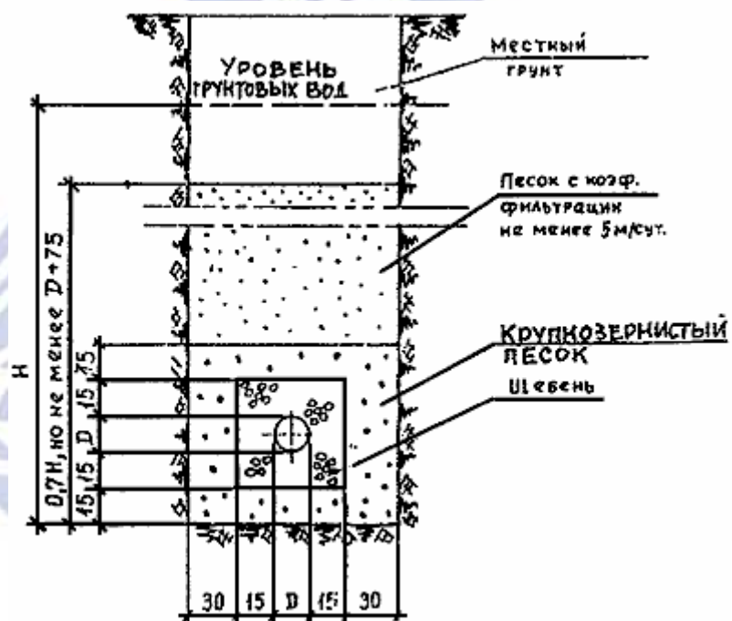
Рис.2. Дренаж несовершенного типа
