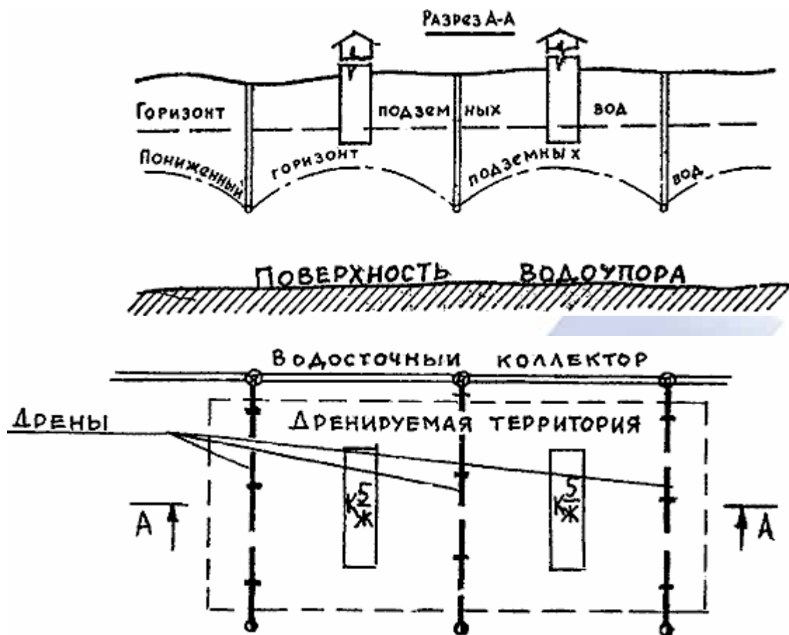
Рис.7. Схема систематического дренажа
