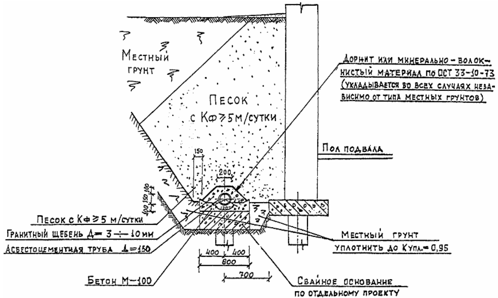
Рис. 15. Пристенный дренаж с применением асбестоцементных труб на свайном основании с засыжкой пазух песком
