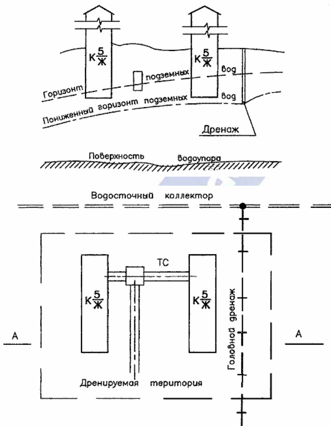
Рис.3. Схема головного дренажа
