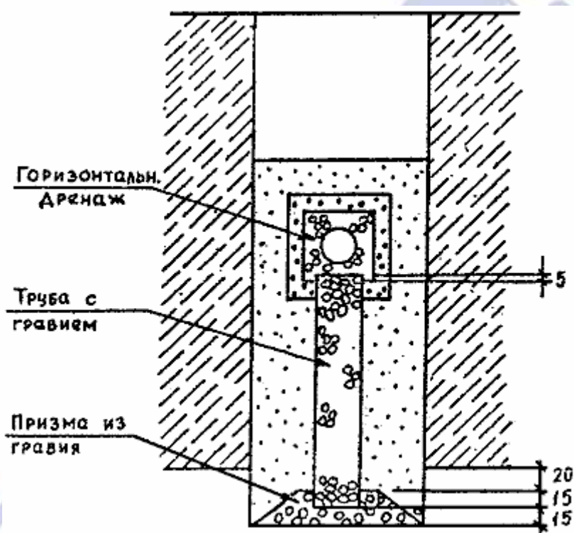
Рис.5. Комбинированный дренаж с вертикальным самоизливающимся колодезем
