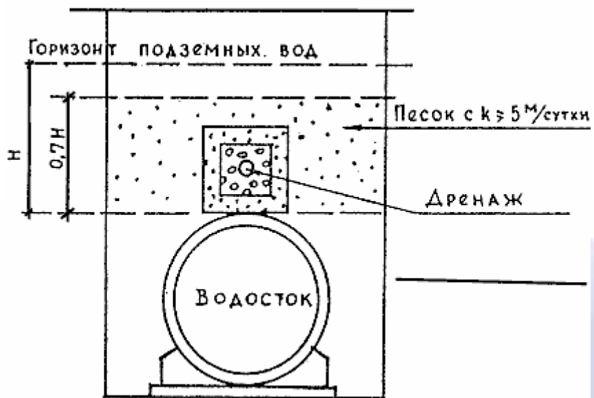
Рис.10. Схема прокладки дренажа над водостоком
