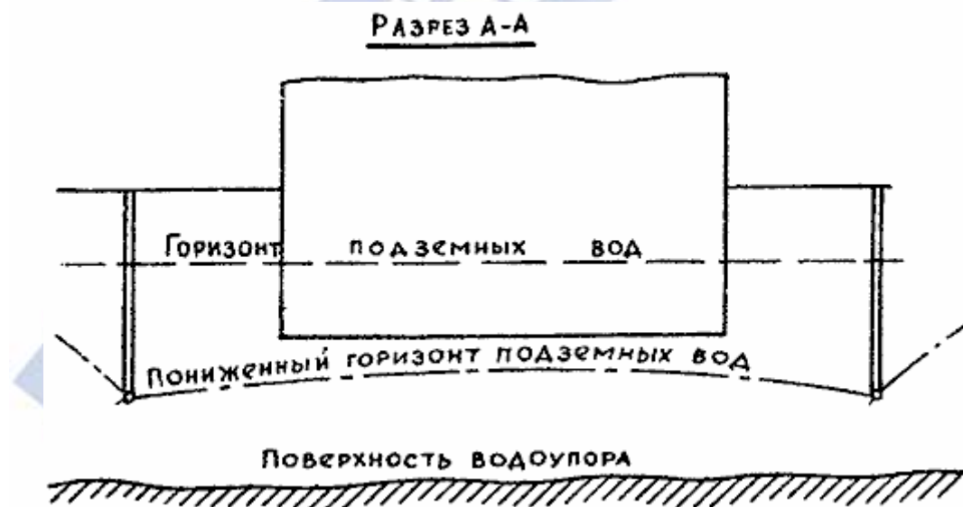
Рис.7. Схема систематического дренажа
