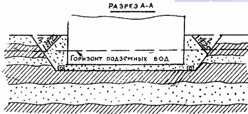
Рис.8. Схема кольцевого дренажа
