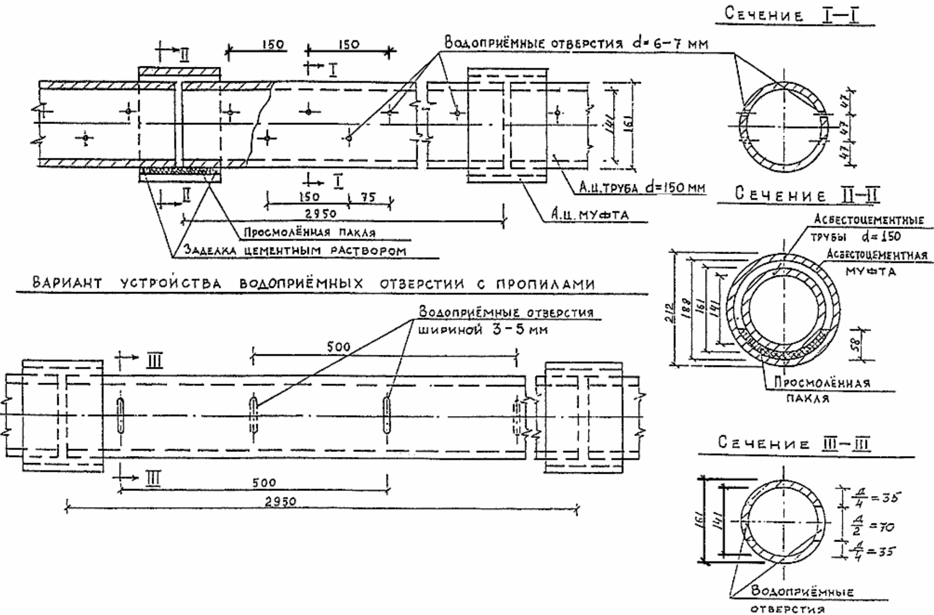
Рис.11. Труба асбестоцементная с водоприёмными отверстиями и с заделкой стыков
